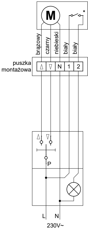
Rys. 25 Schemat połączeń w siłowniku E
