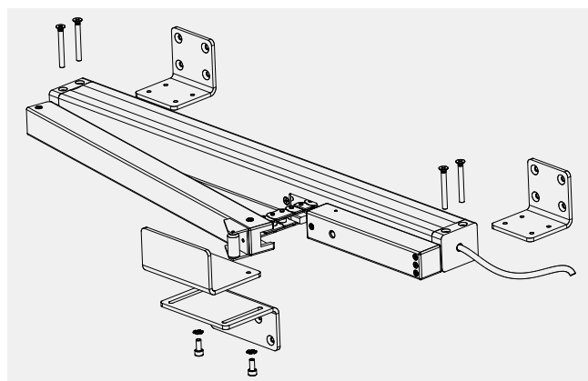
Rys. 44 Zestaw konsol – otwieranie do wewnątrz
