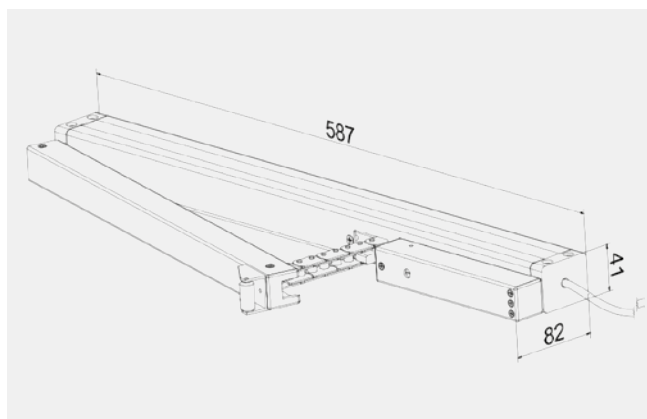
Rys. 43 Wymiary
