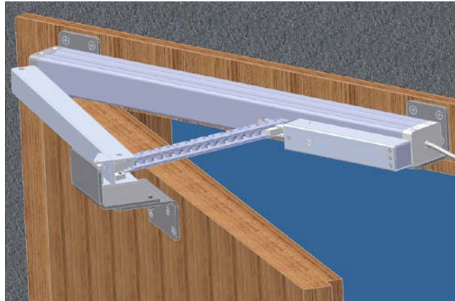
Rys. 46 Otwieranie do wewnątrz
