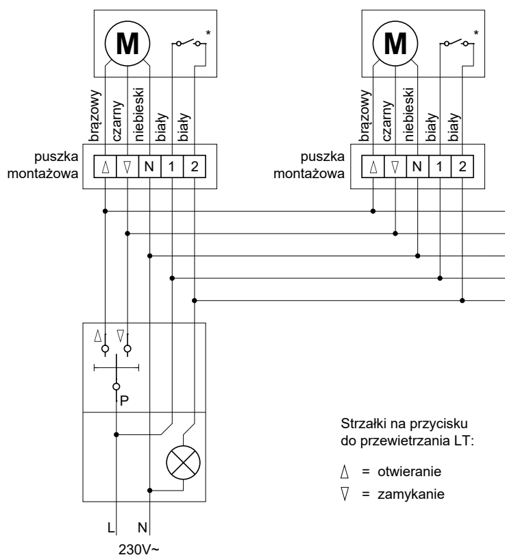
Rys. 33 Schemat połączeń elektrycznego systemu sterowania wentylacją 230 V~
