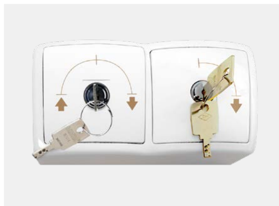
Rys. 32 Łącznik 3- i 2-pozycyjny na kluczyk
