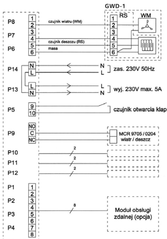
Rys. 22 Schemat podłączeń centrali pogodowej mcr P054 z czujnikami GWD-1
