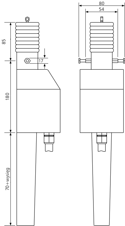
Rys. 24 Wymiary siłownika E
